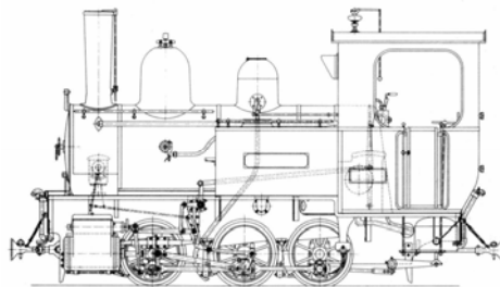
Dampflokomotive der Waldenburgerbahn (heute im VHS Luzern)
